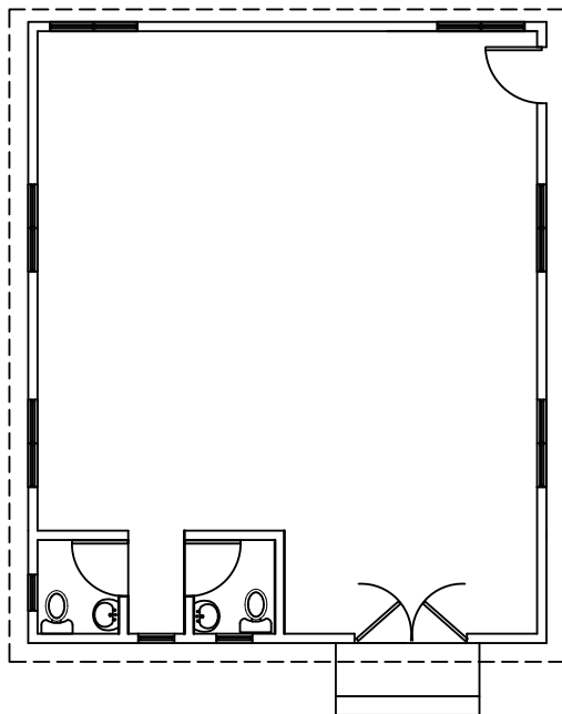
CENTRO COMUNAL PLANTA TIPO B
