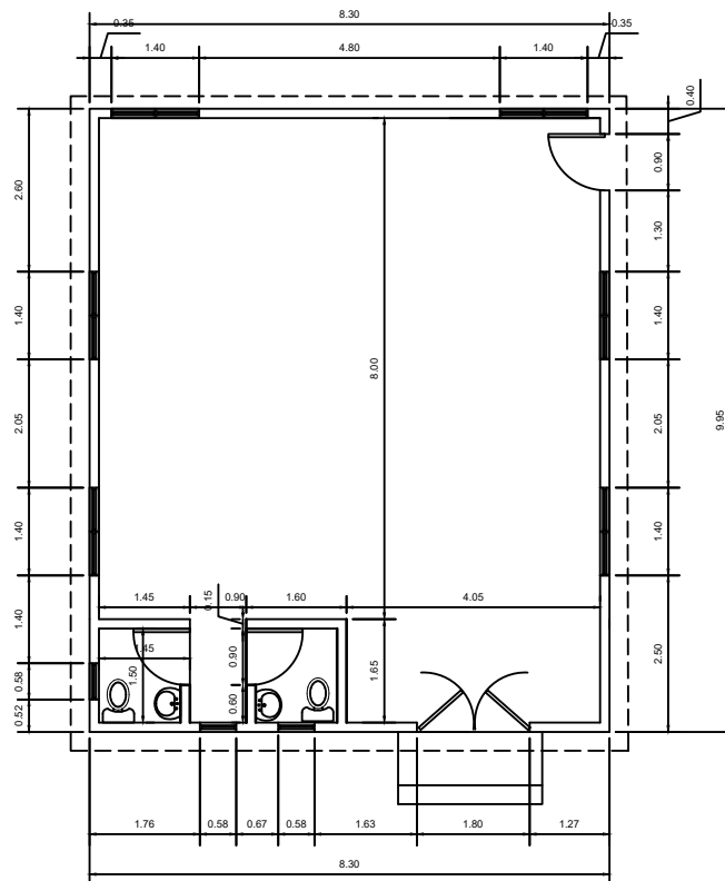
PLANTA DIMENSIONADA
