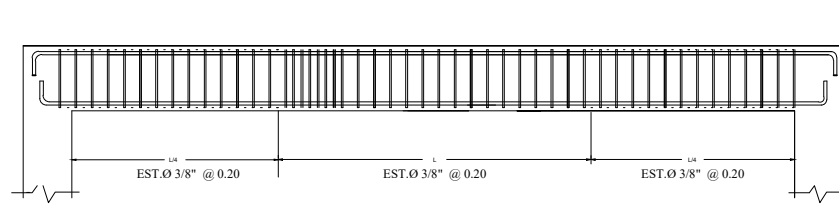
VIGA VP
