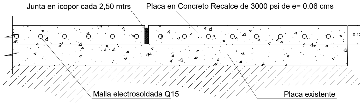
CORTE DE PLACA DE PISO
