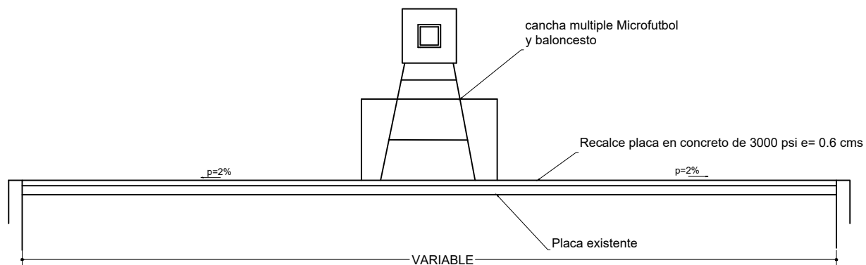
CORTE TRANSVERSAL A- A' ESC: 1:100
